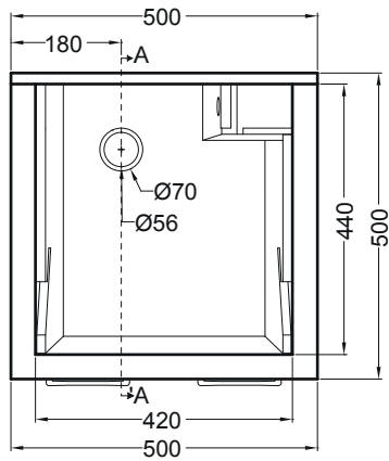
PIANTA
