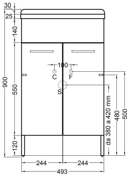
VISTA FRONTALE
